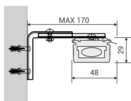
VISTA DI LATO Attacco a parete OPTIONAL
